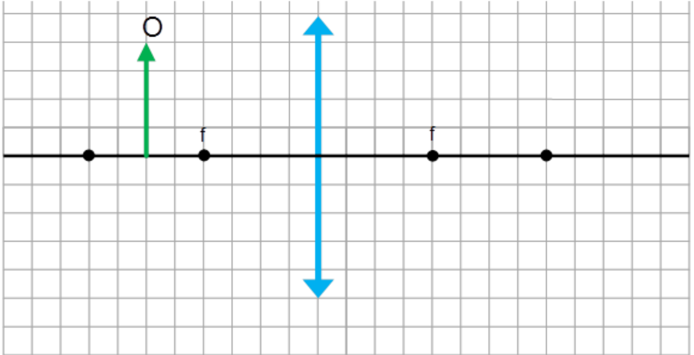
Figura 3: Objeto entre o foco e o anti-principal
